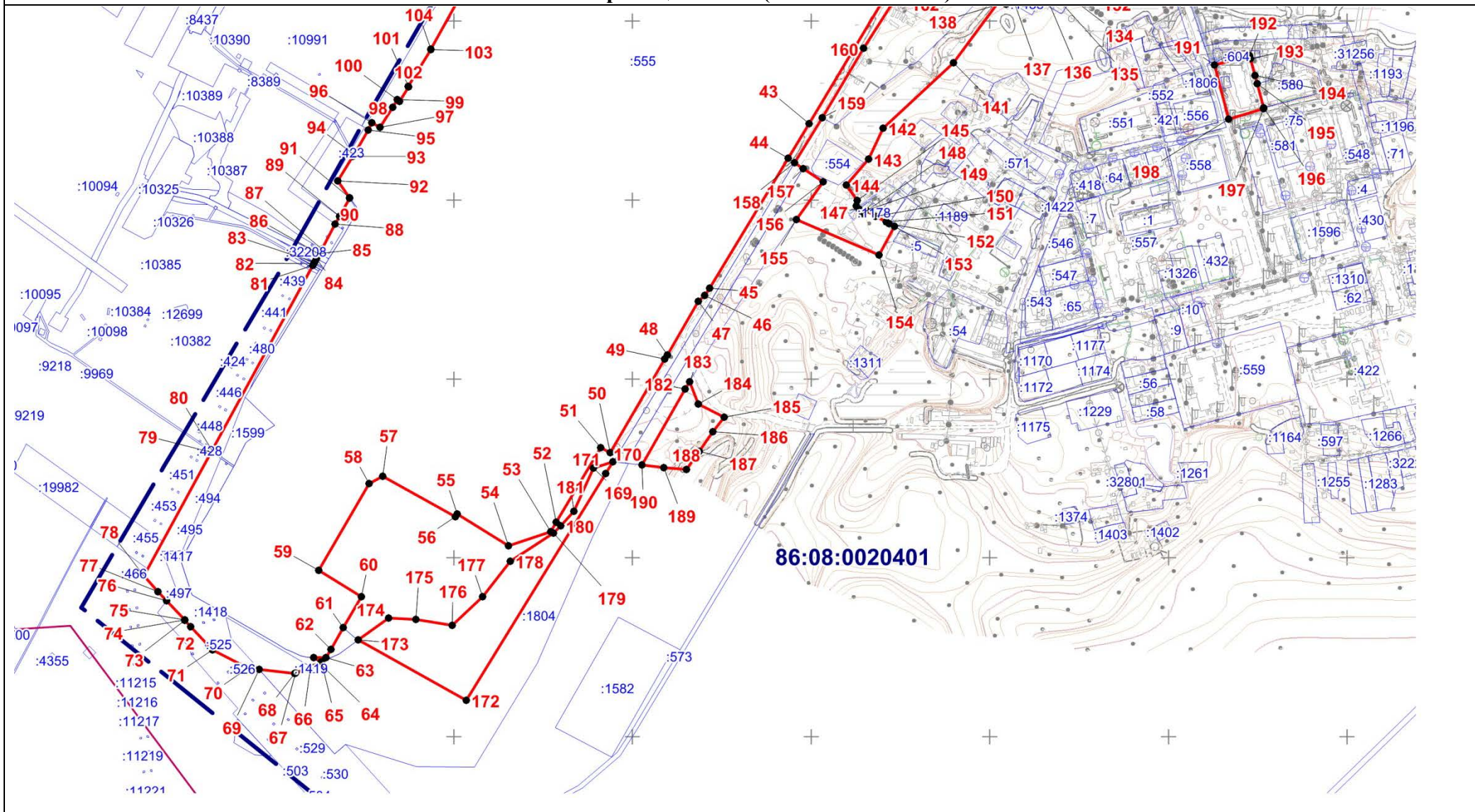
План границ объекта (Выносной лист 2)
