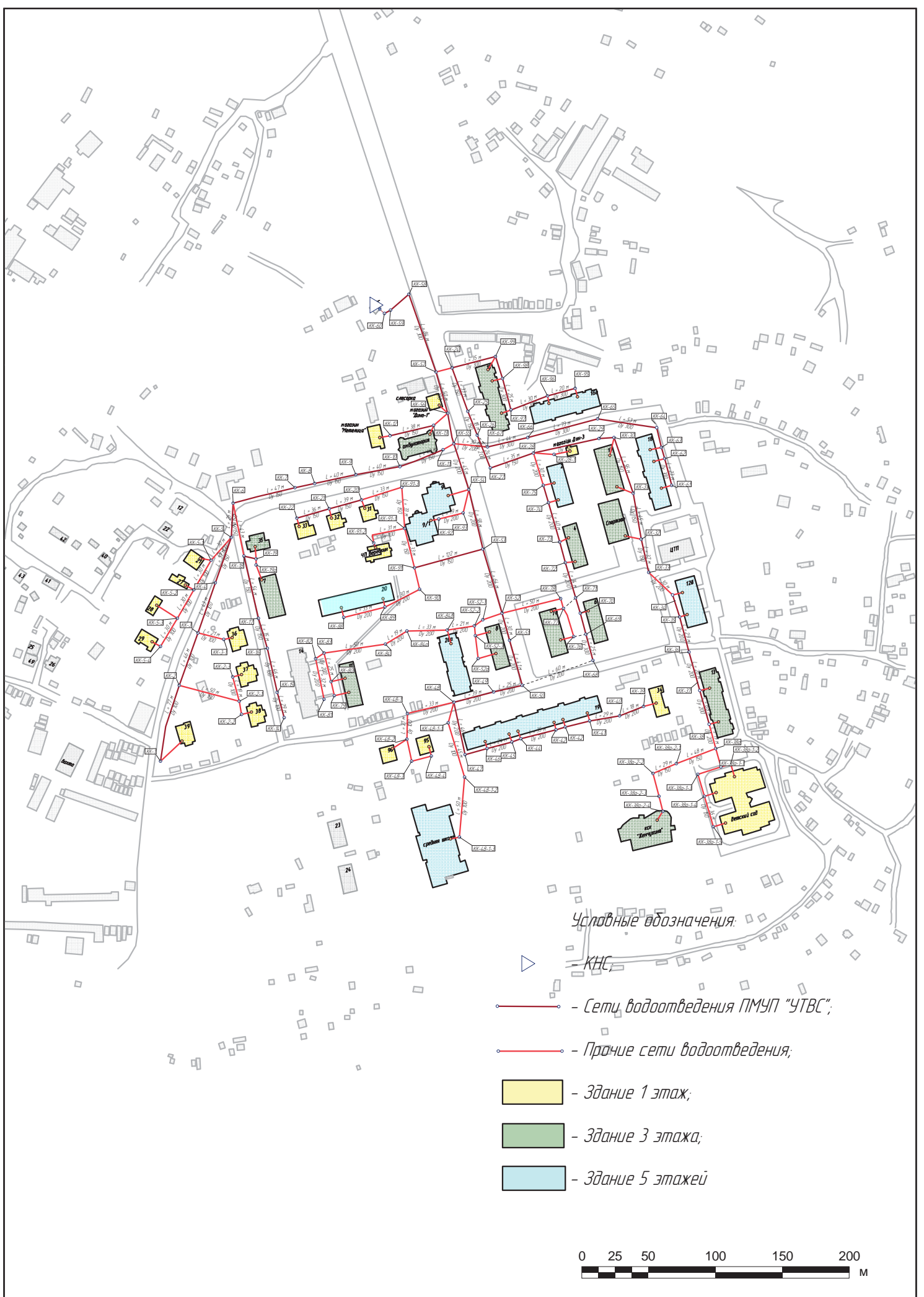
Рисунок 1.4 - Существующая схема сетей водоотведения
